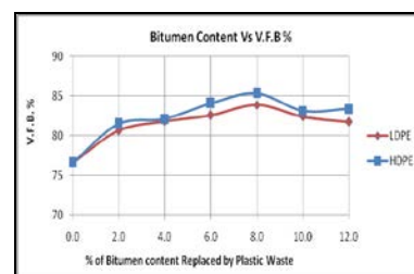
Fig.9 Bitumen Content Vs V.F.B. %
