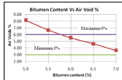
Fig. 3 Bitumen content Vs Air Void %
