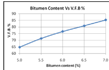
Fig. 4 Bitumen content Vs V.F.B%
